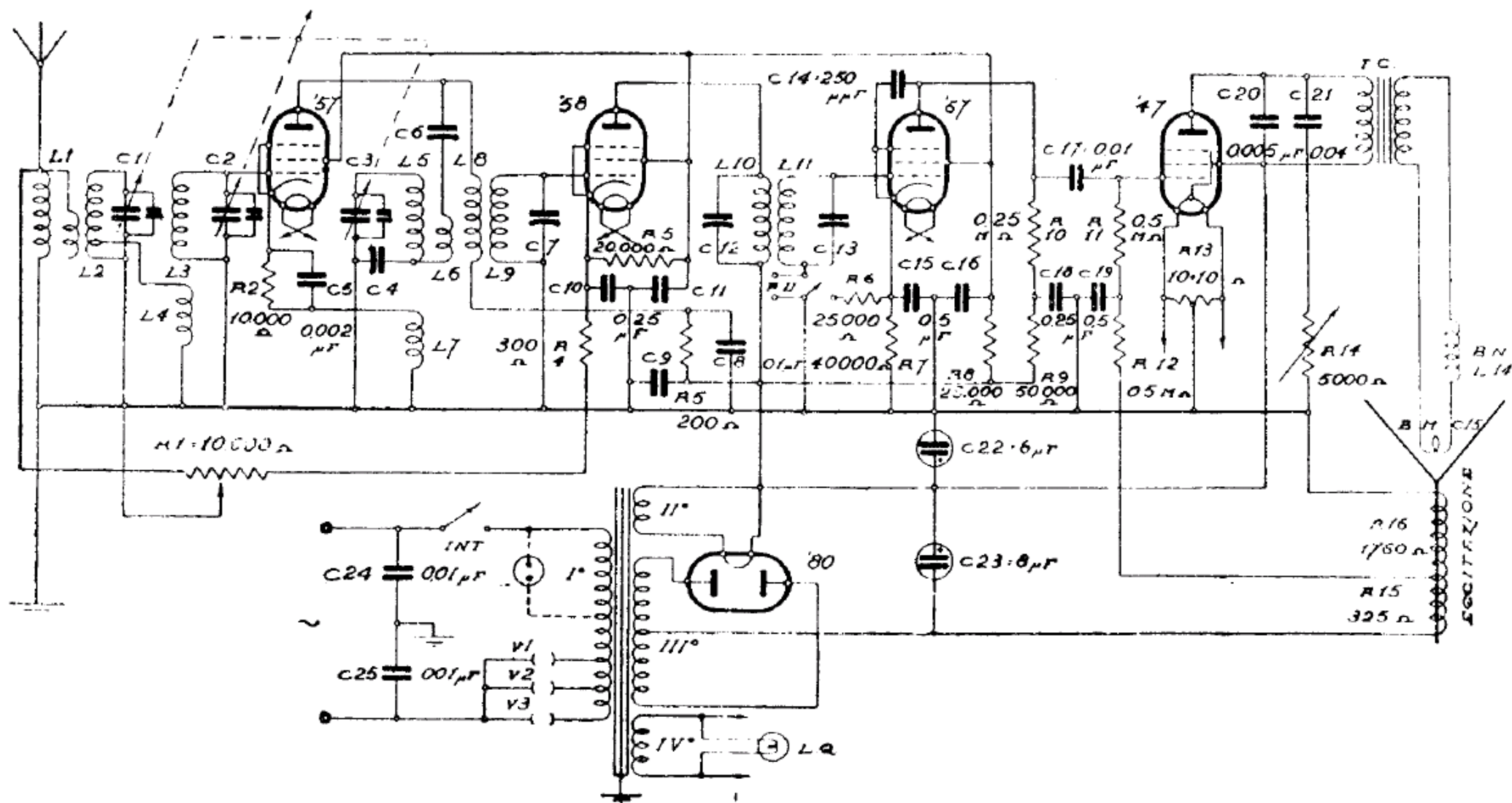
F.I.M.I. - MOD. PHONOLA «581» (ch. 560)
